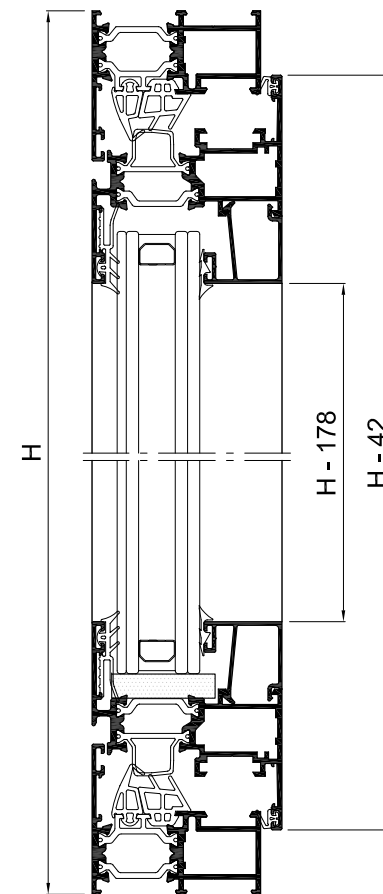
Sección B-B'
