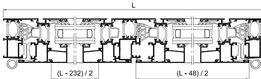
Sección A-A'
